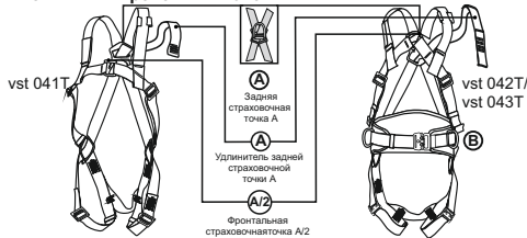
Рис. 2. Типы крепежных точек
