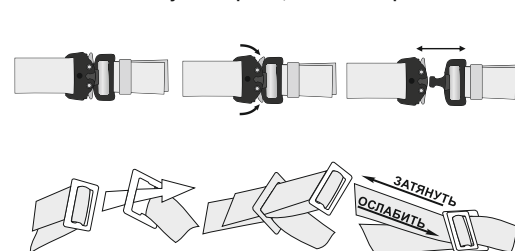
Рис. 6. Типы используемых пряжек, способы заправки
