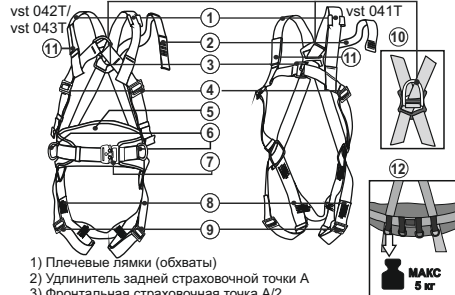
Рис. 1. Внешний вид, составные части и параметры
